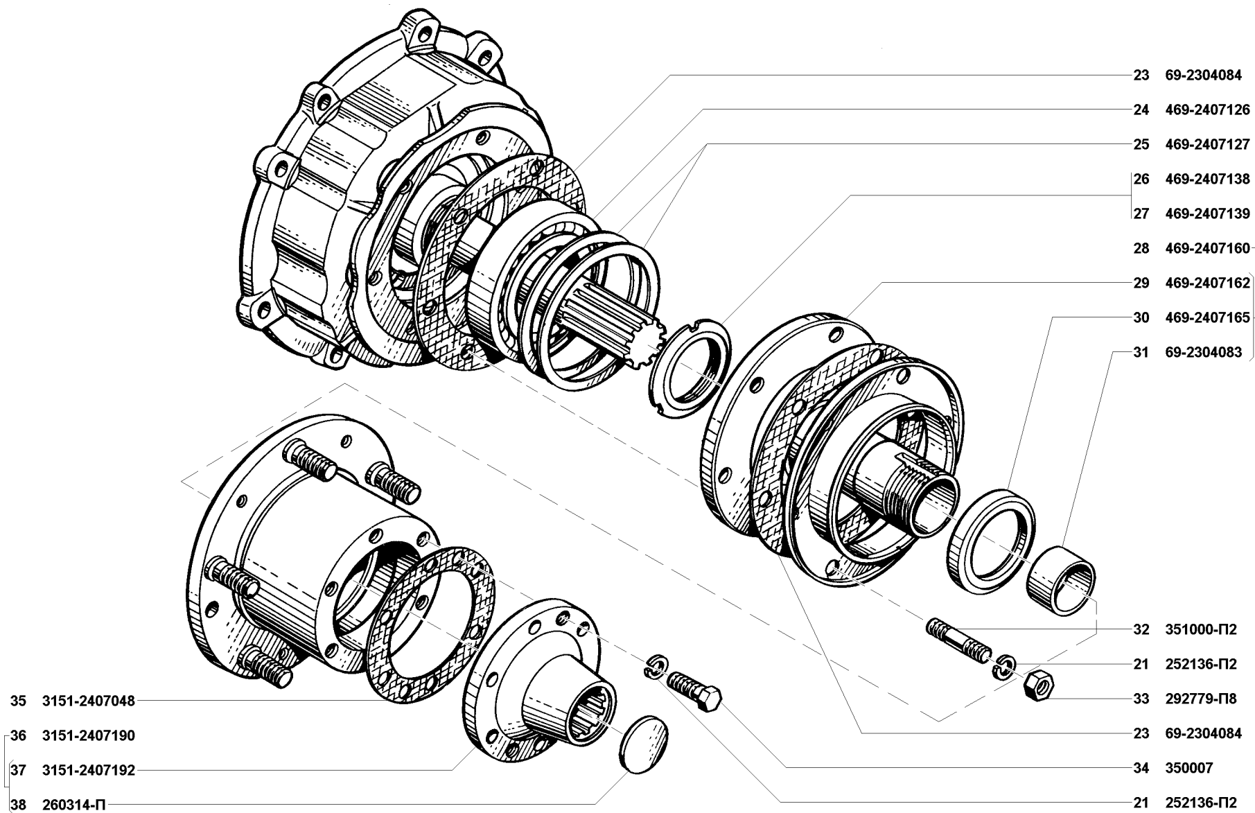
Рис. 80. Редуктор колесный заднего моста (2407)/2
